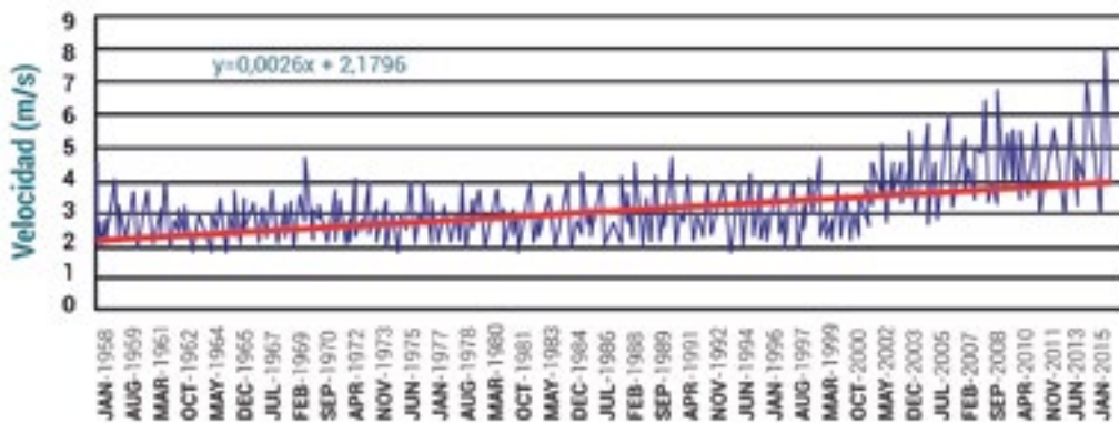
Figura 6. Serie histórica WHOI de la velocidad del viento (84,5°O, 9,5°N).
