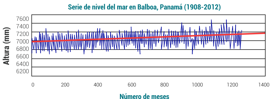
Figura 5. Variación del nivel del mar en Balboa, Panamá.
