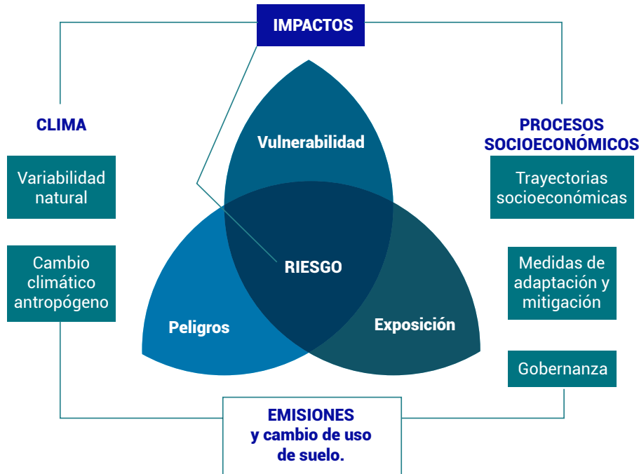
Figura 18. Conceptos relacionados con el riesgo de los impactos conexos al clima (IPCC, 2014).
